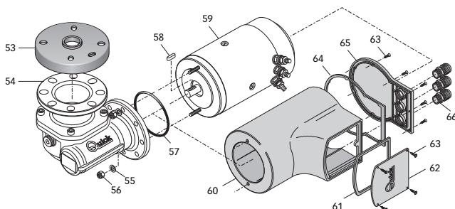
UNTERSETZUNGSGETRIEBE 700/1000W
