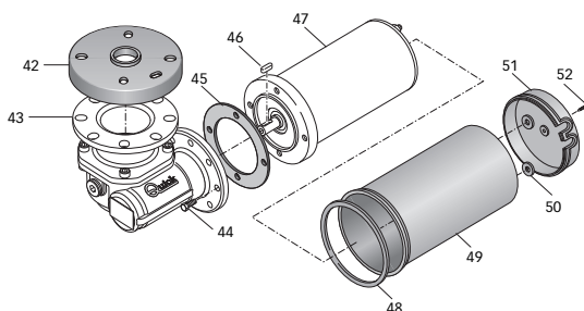
UNTERSETZUNGSGETRIEBE 300/500W
